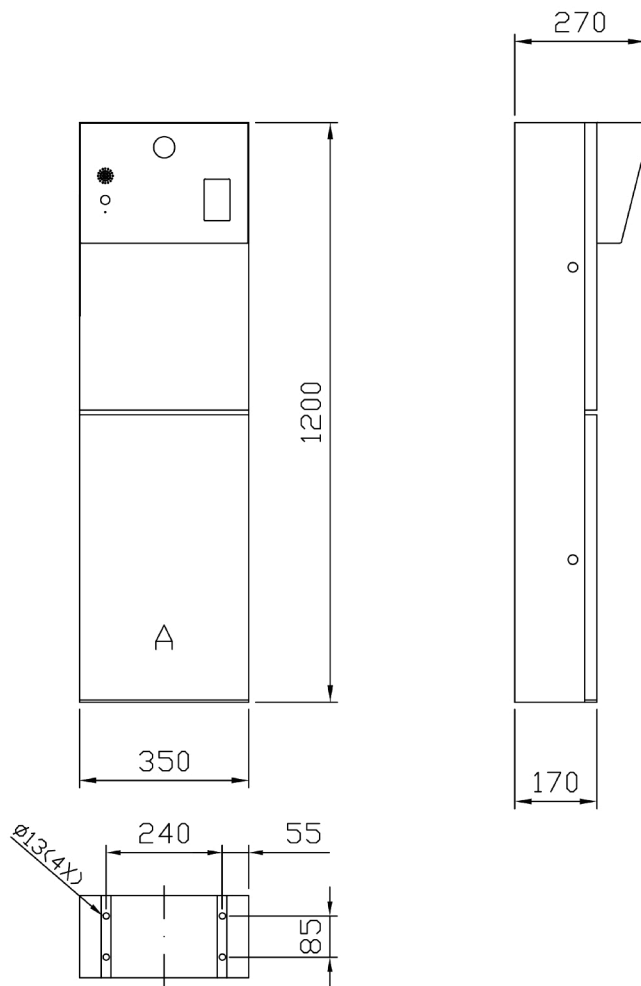
Vista por "A" Detalhe de Fixação
